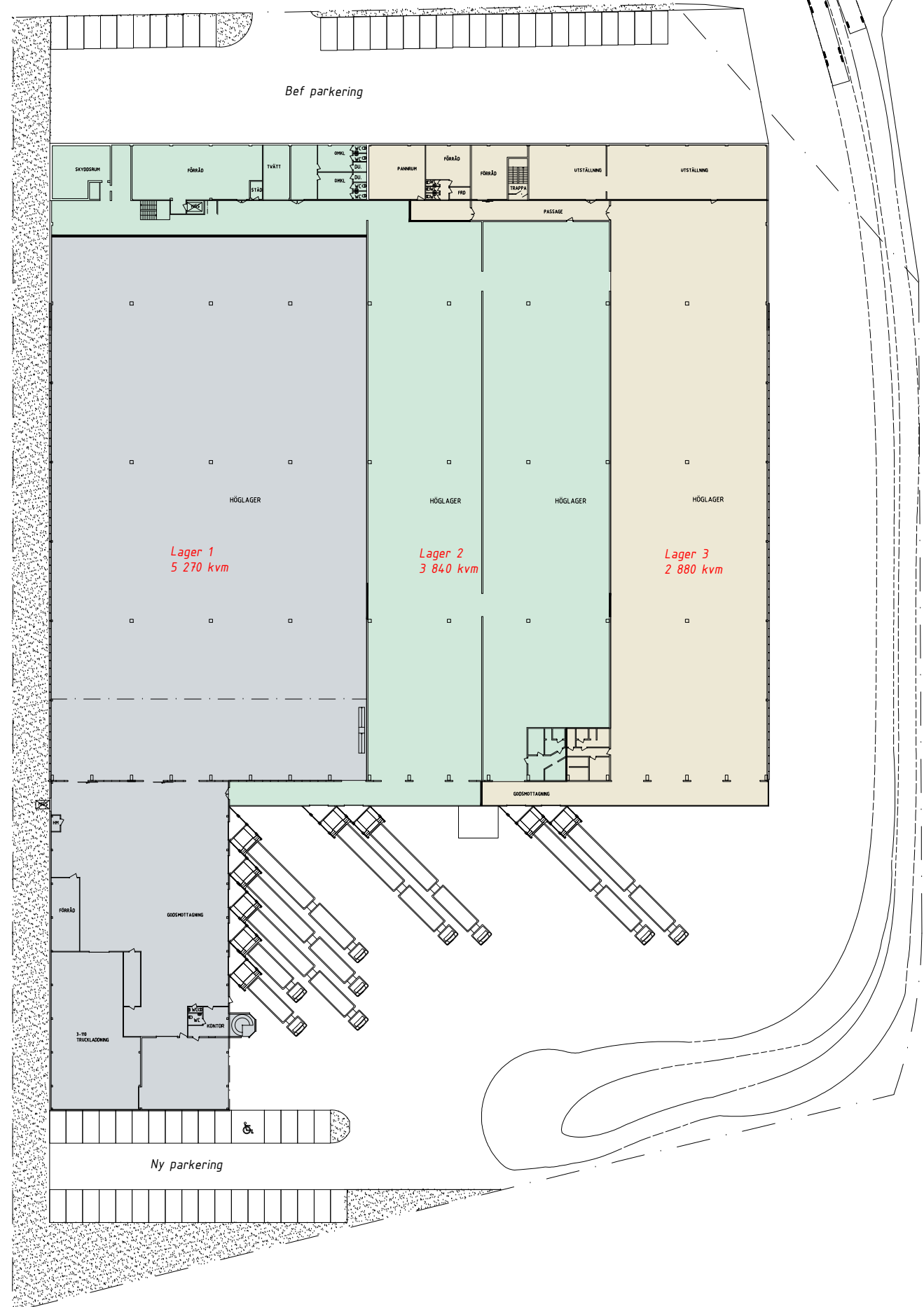
Översiktsplan plan 1 1:400
